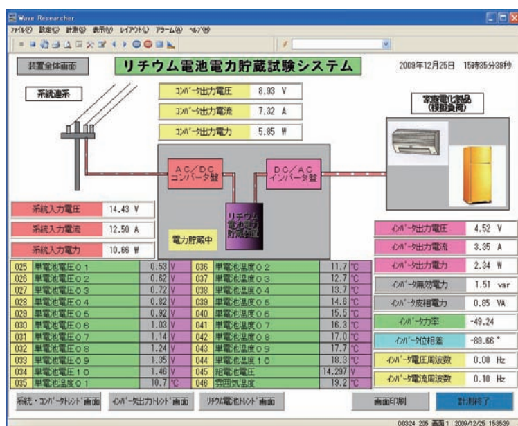
リチウム電池電力貯蔵システム画面表示例
